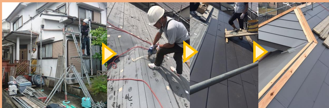
ガルバリウム 鋼板施工
